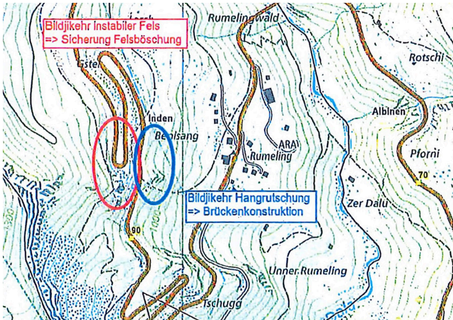
Beilage 1: Standorte Sondierbohrungen
